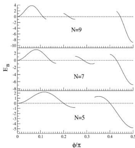
شکل ۲: انرژی پیوند حالت سالیتون N -ذره‌ای برحسب \phi برای سه مقدار مختلف N [۴].
